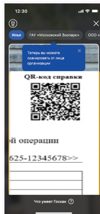
Рисунок 36 – Проверка QR-кода
