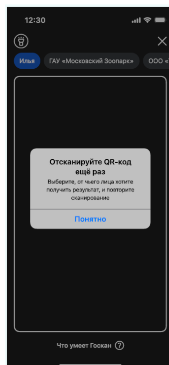
Рисунок 35 – Экран сканирования
